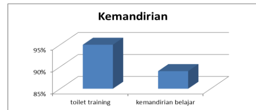
Gambar 4. Diagram Kemandirian
